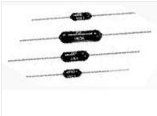
TE 产品编号9-1879678-4 H4 1K0 0.1% 50PPM
