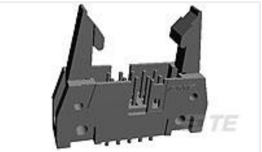
TE 产品编号6364106-4 A/L UNIV HDR 20P VERT LAT
