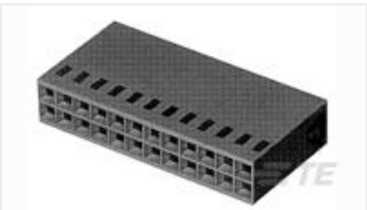
TE 产品编号1-87456-1 16 MODIV HSG COMP DR .100CL
