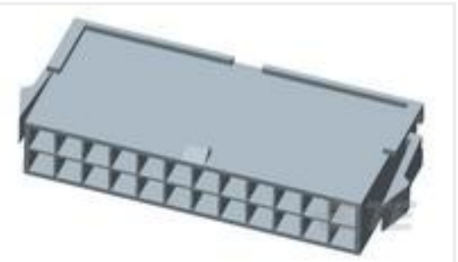
TE 产品编号1-1969613-0 10P PM PLUG VAL-U-LOK V0
