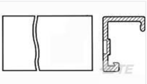
TE 产品编号1-640551-0 10P MTA156 COVER
