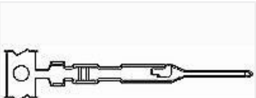
TE 产品编号1-104505-0 MTE PIN 22-26 AWG PLTD
