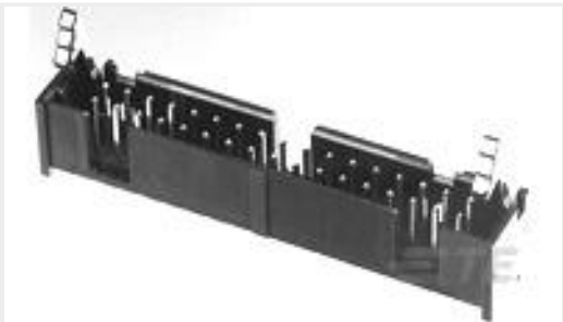
TE 产品编号1761608-9 IDC LOW PRO HDR 26P VERT SHT LAT BLK
