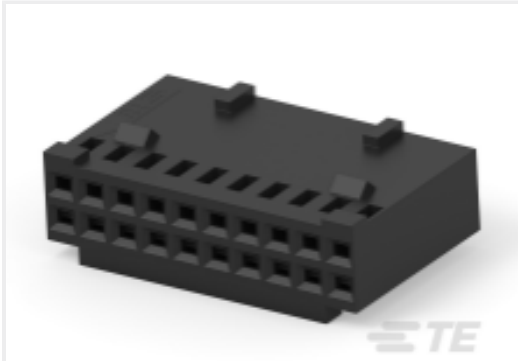
TE 产品编号 1-87631-5 20 MODIV HSG COMP DR .100 POL
