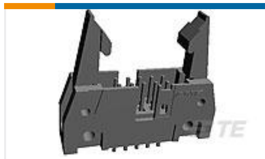
TE 产品编号5102321-4 A/L UNIV HDR 20P VERT LG LAT
