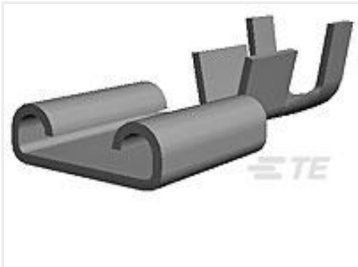
TE 产品编号5-160506-1 250 FASTON REC 20-16 AWG BR
