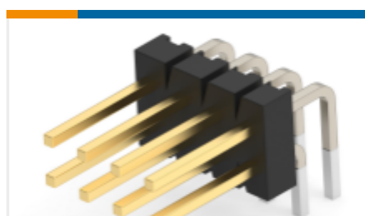
TE 产品编号 5-146309-4 08 MODII HDR DRRR B/A .100CL
