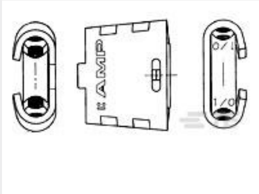
TE 产品编号83592-2 MINIWEDGE,SYM,1/0-#2,CORE
