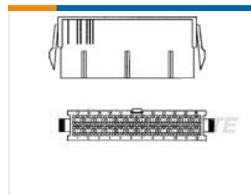
TE 产品编号1-794953-4 14P PM PLUG VAL-U-LOK V2
