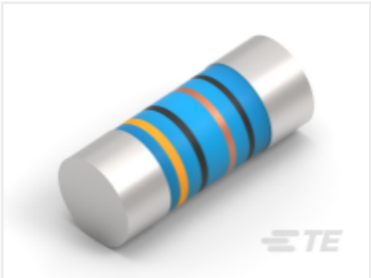
TE 产品编号3-2176315-2 MELF SMA_A 39K 0.1% 15PPM 0204 0.4W
