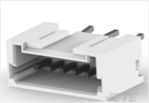
TE 产品编号2-292207-6 MINI CT SGL DIP V 6P BLACK
