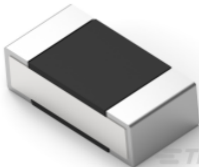
TE 产品编号2-2176308-1 RP 1E 0.1W 215K 0.1% 25PPM 5K RL
