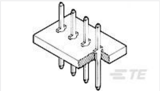
TE 产品编号3-86147-7 MOD I POST PLTD SN
