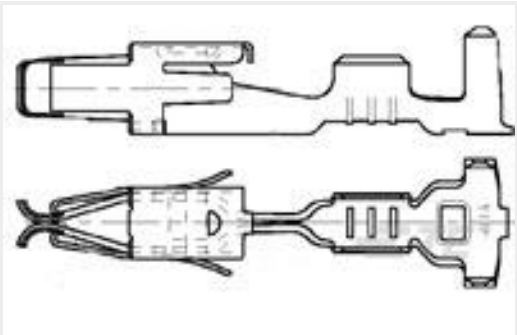
TE 产品编号185026-1 JPT F REC 2.8 Contact SWS Sn
