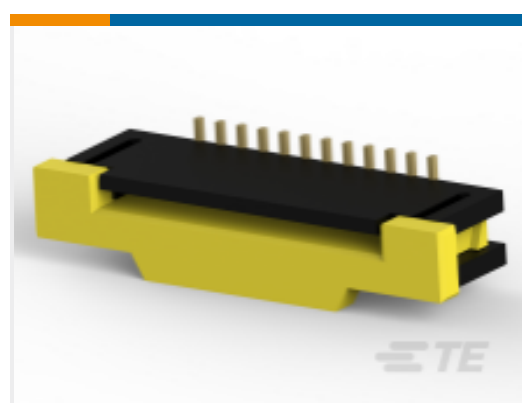
TE 产品编号 1-1734248-2 1.0 FPC, ZIF V/T, SMT, 12P
