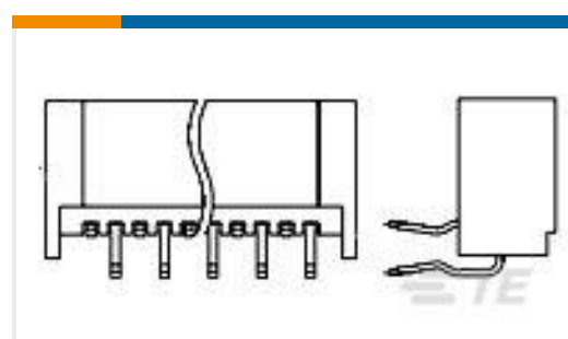
TE 产品编号 1-1734803-7 FPC Non Zif 1.25mm 17P R/A
