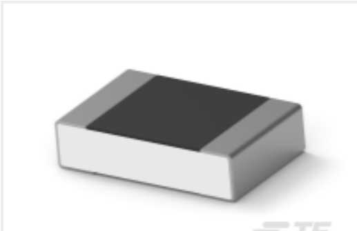
TE 产品编号8-2176379-2 RQ 0805 750R 0.1% 10PPM 5K RL
