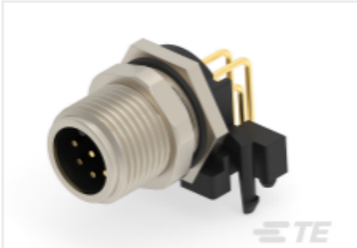
TE 产品编号 T4144015081-000 M12 RA PCB CONN. Male 8 P UN SHIELD
