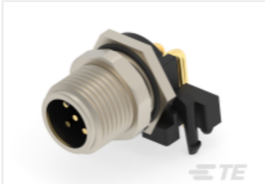
TE 产品编号 T4144015051-000 M12 R/A M PNL REAR A-CODE 5P PCBSTD
