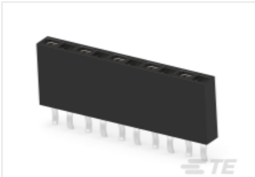
TE 产品编号 1-215299-0 10P HV100 REC CON. TE, 8.5MM
