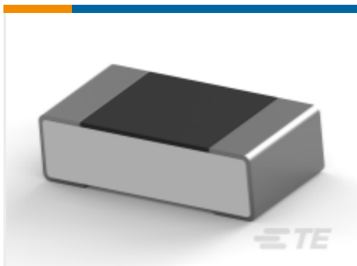
TE 产品编号1-2176367-9 RQ 0603 7K15 0.1% 10PPM 1K RL
