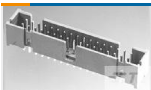
TE 产品编号5104338-2 A/L LOW PRO HDR 14P VERT HT
