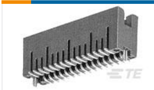
TE 产品编号5-104656-5 50 50/50 HDR DRST SFMNT.320 SN
