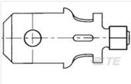
TE 产品编号60284-2 205 FASTON TAB TPBR
