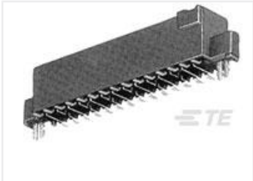
TE 产品编号6-104652-0 100 50/50 GRID DRST SFMNT RCPT
