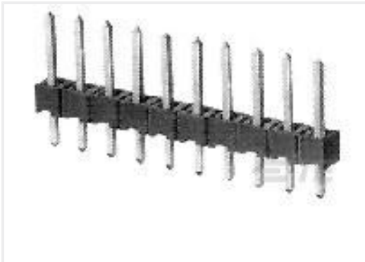
TE 产品编号826936-6 6P AMPMODU II STIFT LEI
