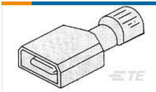
TE 产品编号3-521142-2 ULTRA-FAST 250 ASY TAB 16-14 AWG TPBR
