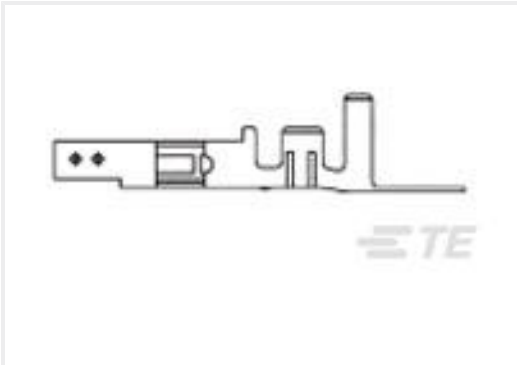
TE 产品编号794956-3 VAL-U-LOK SKT PHBZ SN 22-18AWG
