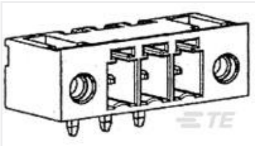
TE 产品编号284541-6 6 POS TERMI-BLOK 900 SF 3,81 m
