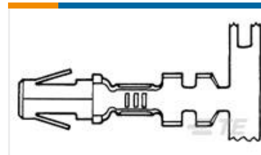
TE 产品编号350390-1 .140 DIA SOK 14-10 PTPBR L/P
