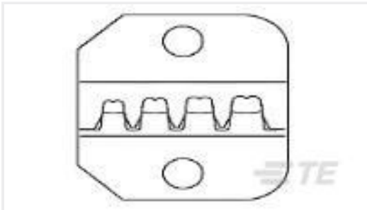
TE 产品编号58509-1 PRO-CRIMPER DIE BUDGET
