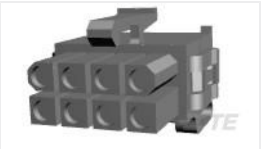
TE 产品编号794245-1 08P MINI UMNL2 PLUG HSG UL94V2
