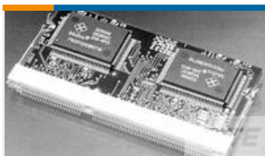
TE 产品编号390113-1 SKT,SODIMM,144P,SDRAM3.3V,STD, TY-S
