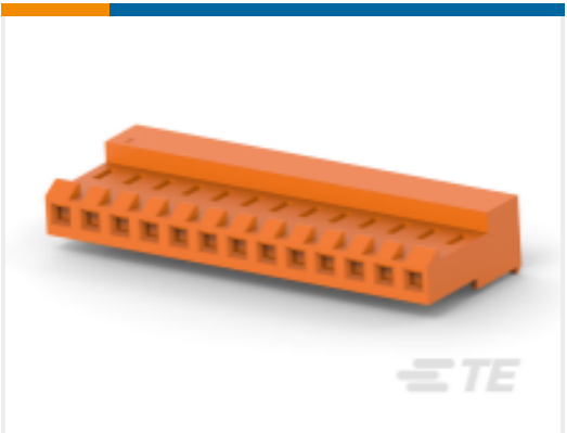
TE 产品编号 4-641148-3 13P MTA156 ASSY 18AWG ORA LF
