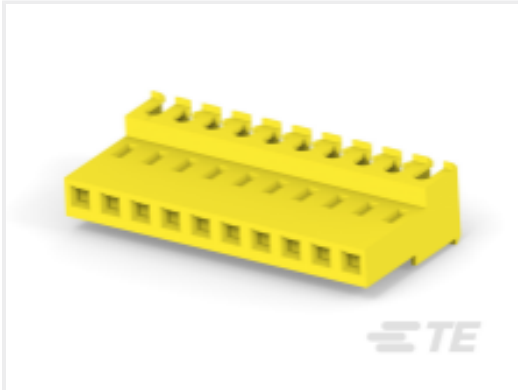
TE 产品编号 4-640605-0 10P MTA156 CONN ASSY 20AWG LF
