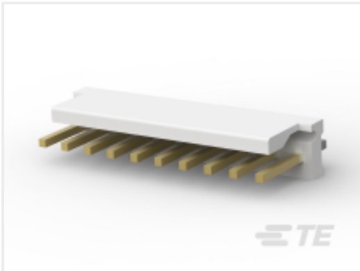
TE 产品编号 4-641208-0 10P MTA156 HDR ASSY FL ST LF
