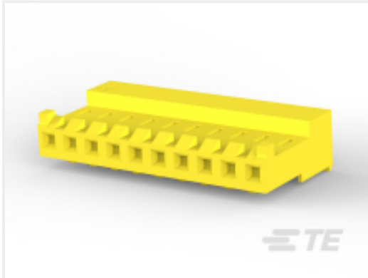
TE 产品编号 4-644663-0 10P MTA156 CONN ASSY 20AWG LF
