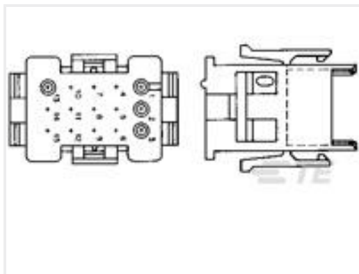
TE 产品编号1-640513-0 15P MR II CAP HSG V0
