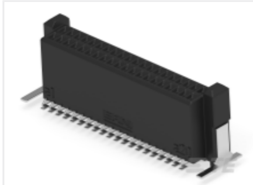
TE 产品编号294017-E DRCB 0,80 40 F SMD F6 137 E009 094 GU-H
