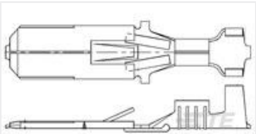
TE 产品编号280081-2 FF 250 TAB 0.8-2MM2 TPBR
