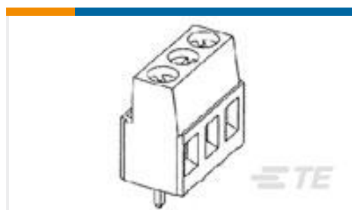
TE 产品编号796949-9 9 POS TERMI-BLOK PCB MOUNT
