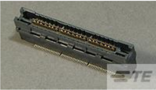
TE 产品编号 5767094-3 MICT,RECPT,114,ASY,PDNI,EXTD
