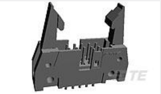
TE 产品编号3-5499206-0 A/L UNIV HDR 50P VERT LAT B
