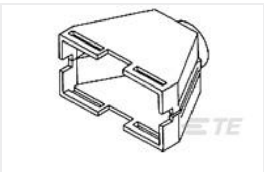
TE 产品编号480594-1 36P STR/REL HSG HNGD V0
