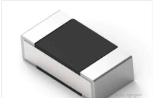
TE 产品编号2-2176305-5 RP 1E 0.1W 191R 0.1% 25PPM 5K RL
