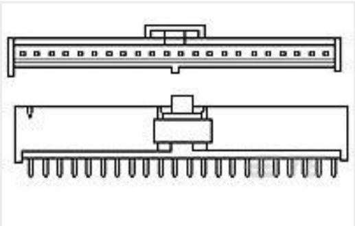
TE 产品编号1888291-1 FPH-0421G=FLXPAC HDR P 04 ST LF
