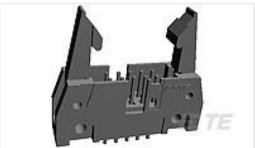
TE 产品编号5499922-6 A/L UNIV HDR 26P VERT LAT
