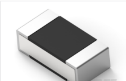
TE 产品编号9-2176306-5 RP 1E 0.1W 11K 0.1% 25PPM 5K RL
