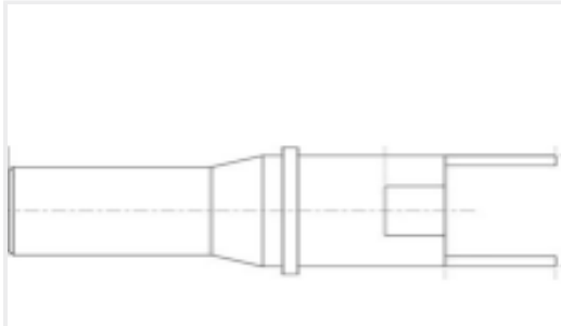
TE 产品编号 1604940-2 SHELL,BLANK,PIN,SZ 8,FR/FR
