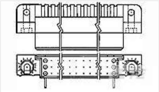
TE 产品编号 532431-3 HDI RECP ASSY 3 ROW 96 POS
